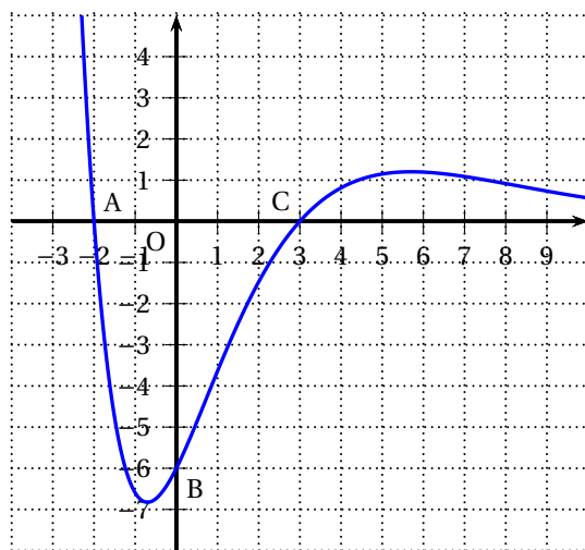
Courbe représentative de la fonction f''
